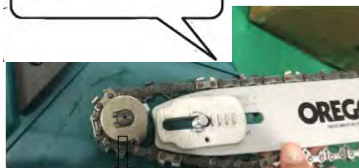
ozubené koliesko
