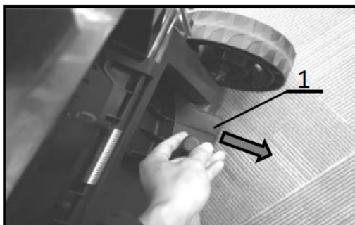
1. Wkładka do mulczowania
