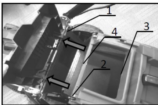
1. Hřídel 2. Háček 3. Sběrný koš 4. Přepážka koše
