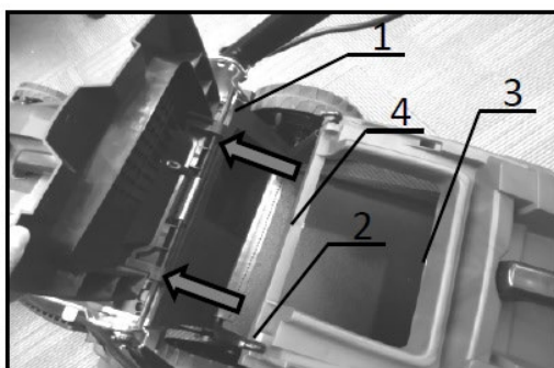
1. Wał 2. Hak 3. Kosz 4. Osłona
